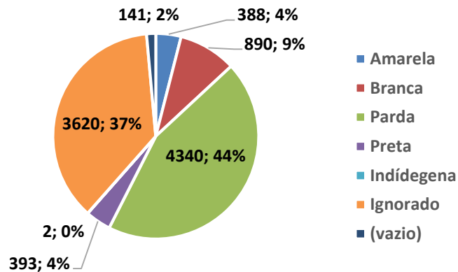
Gráfico 11. Número e Percentual de casos leves confirmados para COVID-19, segundo raça/cor. Cabo de Santo Agostinho, 2020-2022.
